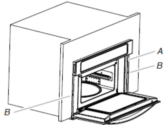
A. Rail de montage B. Vis à tête plate
